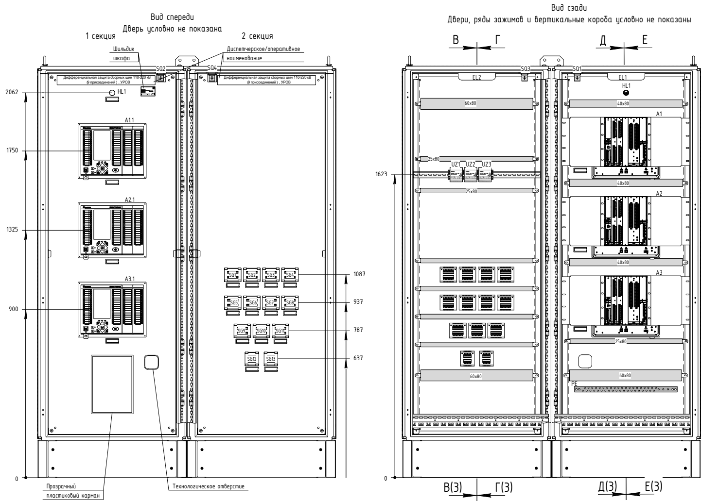
Рисунок Б.2 – Чертеж общего вида (часть 2)
